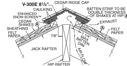
V-300E 8 1/2\"/>
