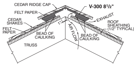
V-300 8 1/2\"/>
