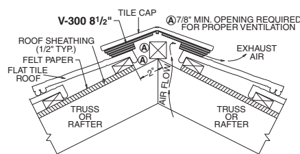
V-300 8 1/2\"/>
